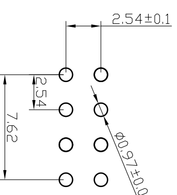
PCB开孔
